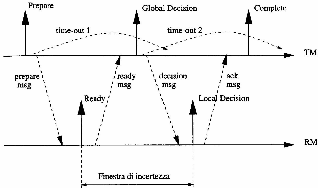
Figura 10.9 Protocollo di commit a due fasi
