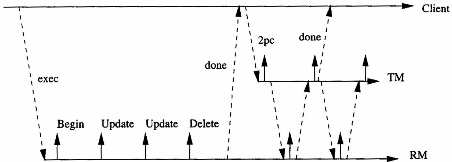
Figura 10.10 Protocollo di commit a due fasi nel contesto di una transazione
