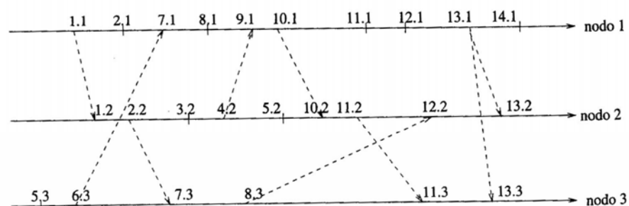
Figura 10.6 Esempio di assegnamento di timestamp col metodo di Lamport
