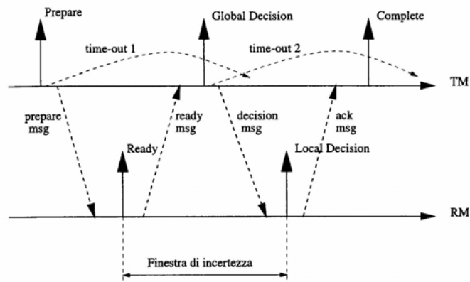
Figura 10.9 Protocollo di commit a due fasi
